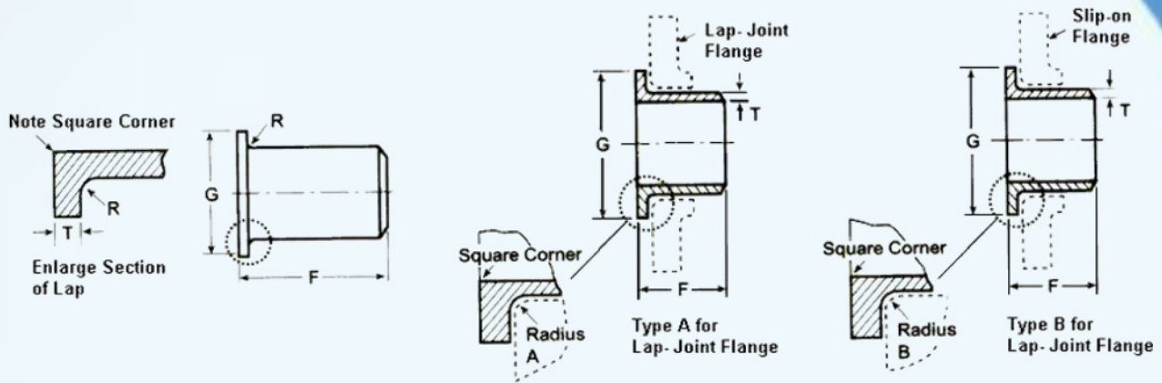
ANSI B16.9
